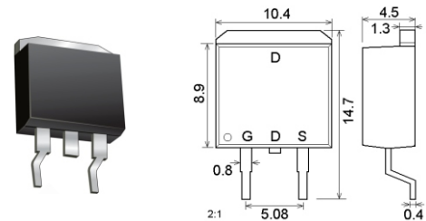
D2PAK / TO263AB
