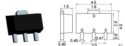
SOT89 / TO243AA
