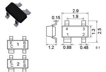
SOT143 / TO253AA
