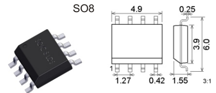
SO8
