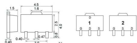
SOT89 / TO243AA
