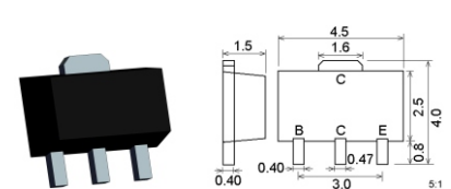
SOT89 / TO243AA
