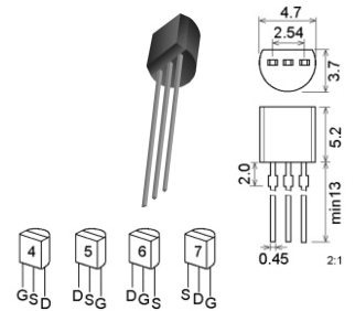
TO92 / SC43 / SOT54
