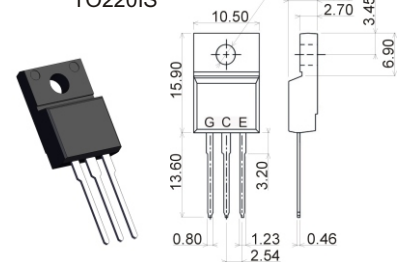
TO220IS
