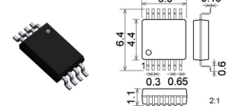
TSSOP8
