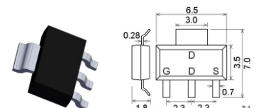
SOT223 / TO261AA
