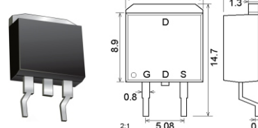
D2PAK / TO263AB
