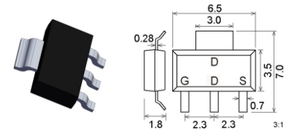
SOT223 / TO261AA
