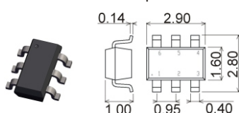
TSOT23-6 / SuperSOT6
