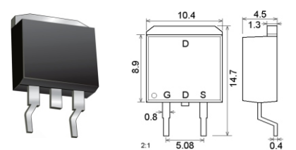
D2PAK / TO263AB
