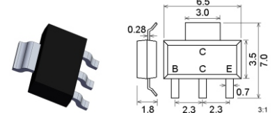
SOT223 / TO261AA
