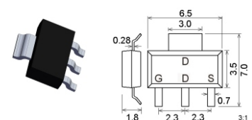
SOT223 / TO261AA
