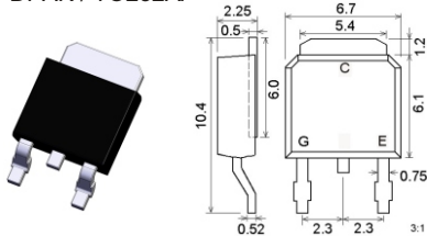
DPAK / TO252AA
