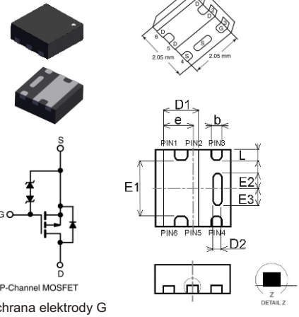
SC-70-6L / PowerPAK
