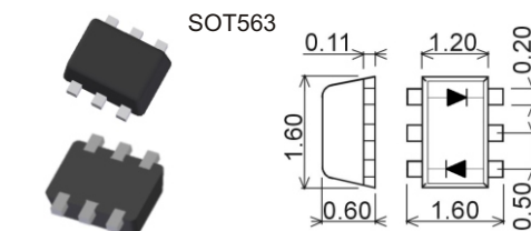
SOT563
