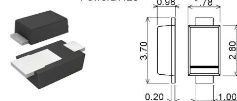
PowerDI123
