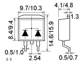
D2PAK (TO263)
